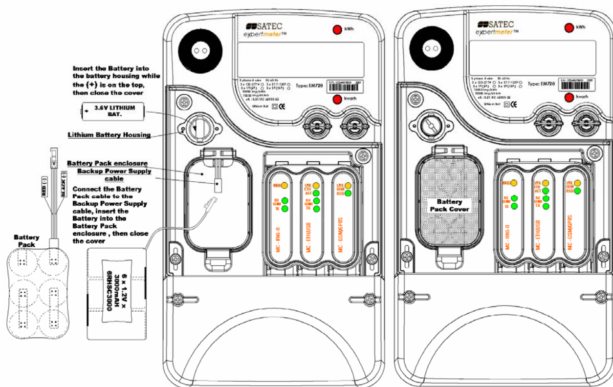
Рис.3 Установка батарей прибора
